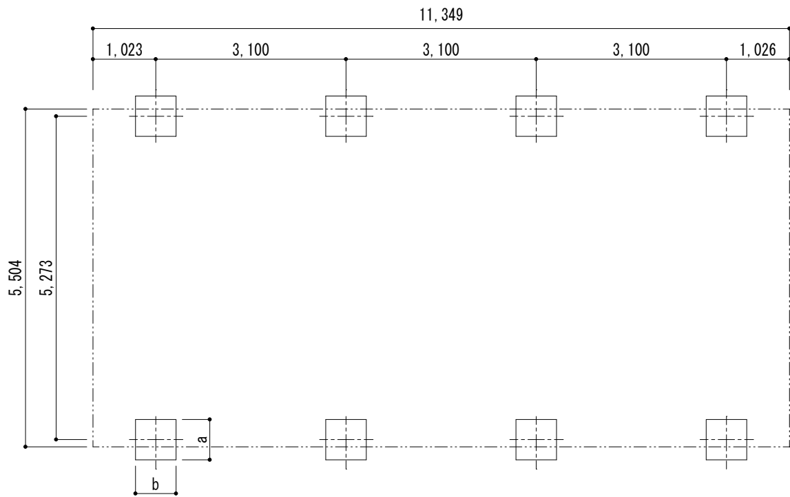
■基礎配置図
